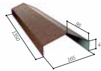
GAŚIOR DŁUGI CORONA AR95
