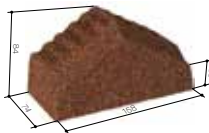
ZAKOŃCZENIE GAŚIORA SENATOR/CORONA
