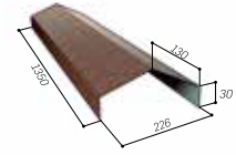
GAŚIOR DŁUGI CORONA AR130
