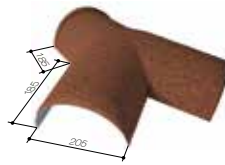
TRÓJNIK GAŚIORA 205 15-30°
