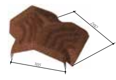
TRÓJNIK GAŚIORA CORONA 15-45°
