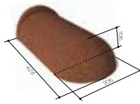
GAŚIOR POCZĄTKOWY 205
