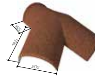
TRÓJNIK GAŚIORA 205 30-45°
